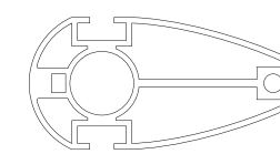
POTEAU OVOIDE
